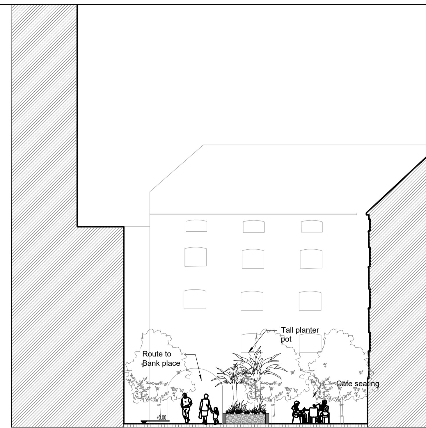
B-B' The Granary SCALE: 1:125
